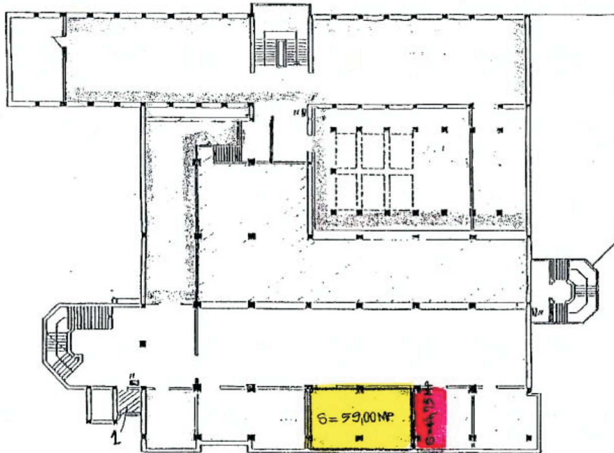
PLAN ETAJ
